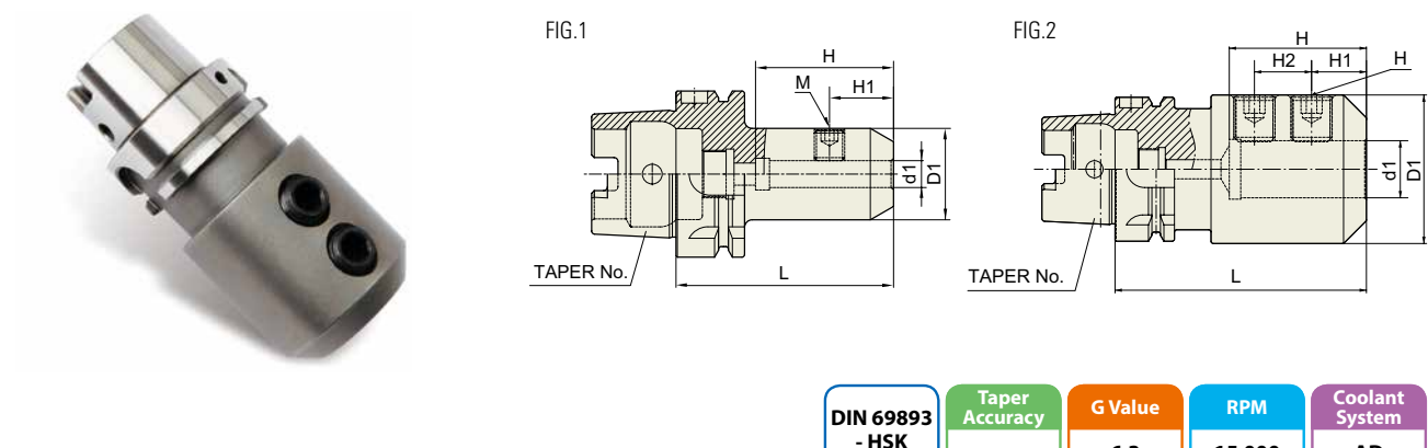
■ DIN 69893/ISO 12164-1-HSK FORM A
